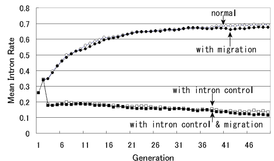
(b) Intron Ratios.
